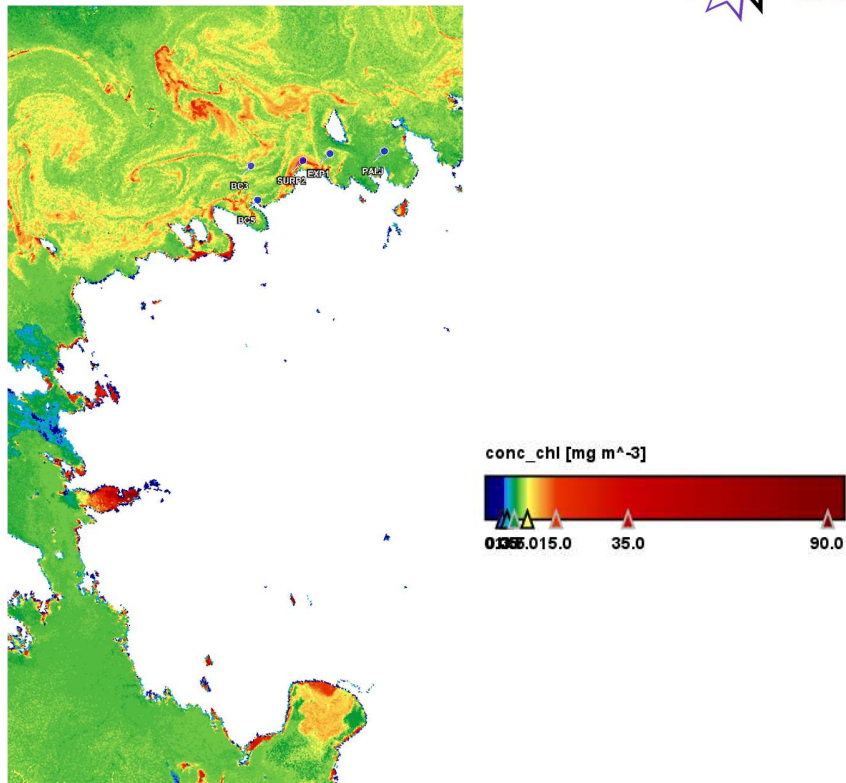
Joonis 1. Eesti rannikumere klorofüllü kontsentratsioon 08.08.2020 Sentinel-3B pildil.
